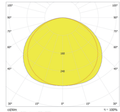
ArcLine Outdoor Mini 18 RGB - Non Optic
