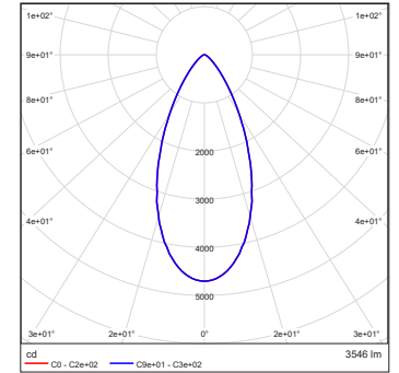
Eminere Inground 4 MC RGBCW Anti-Skid Glass 50dg
