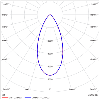
Eminere Inground 4 MC RGBCW Anti-Skid Glass 50dg
