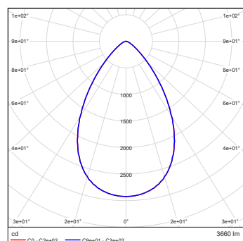
Eminere Inground 4 MC RGBCW Clear Glass 65dq
